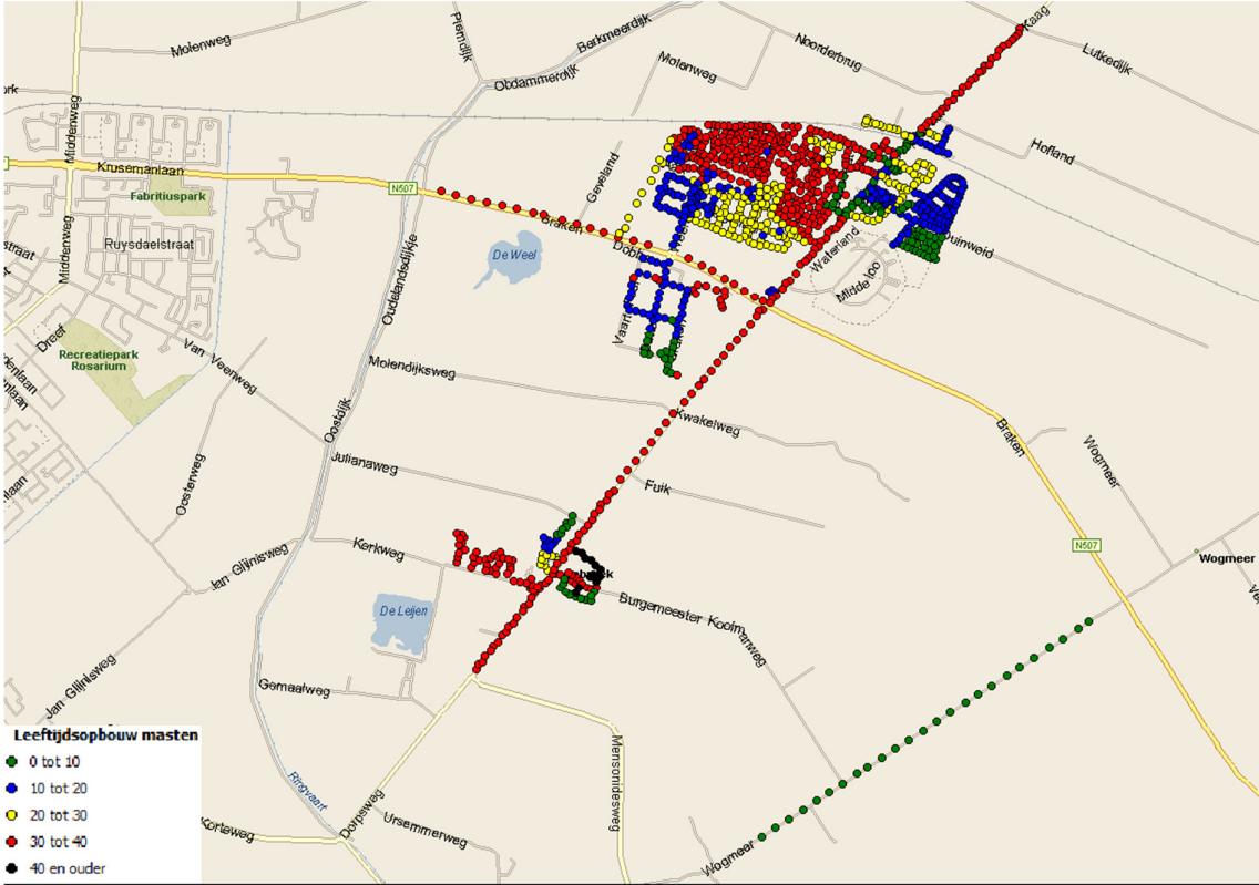
Figuur 9: Leeftijdsopbouw lichtmasten in het noordwestelijke gedeelte van de gemeente Koggenland
