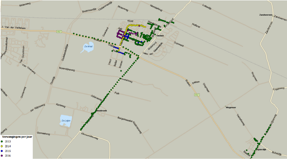
Figuur 15: Vervangingen per jaar in het noordwestelijke gedeelte van de gemeente Koggenland
