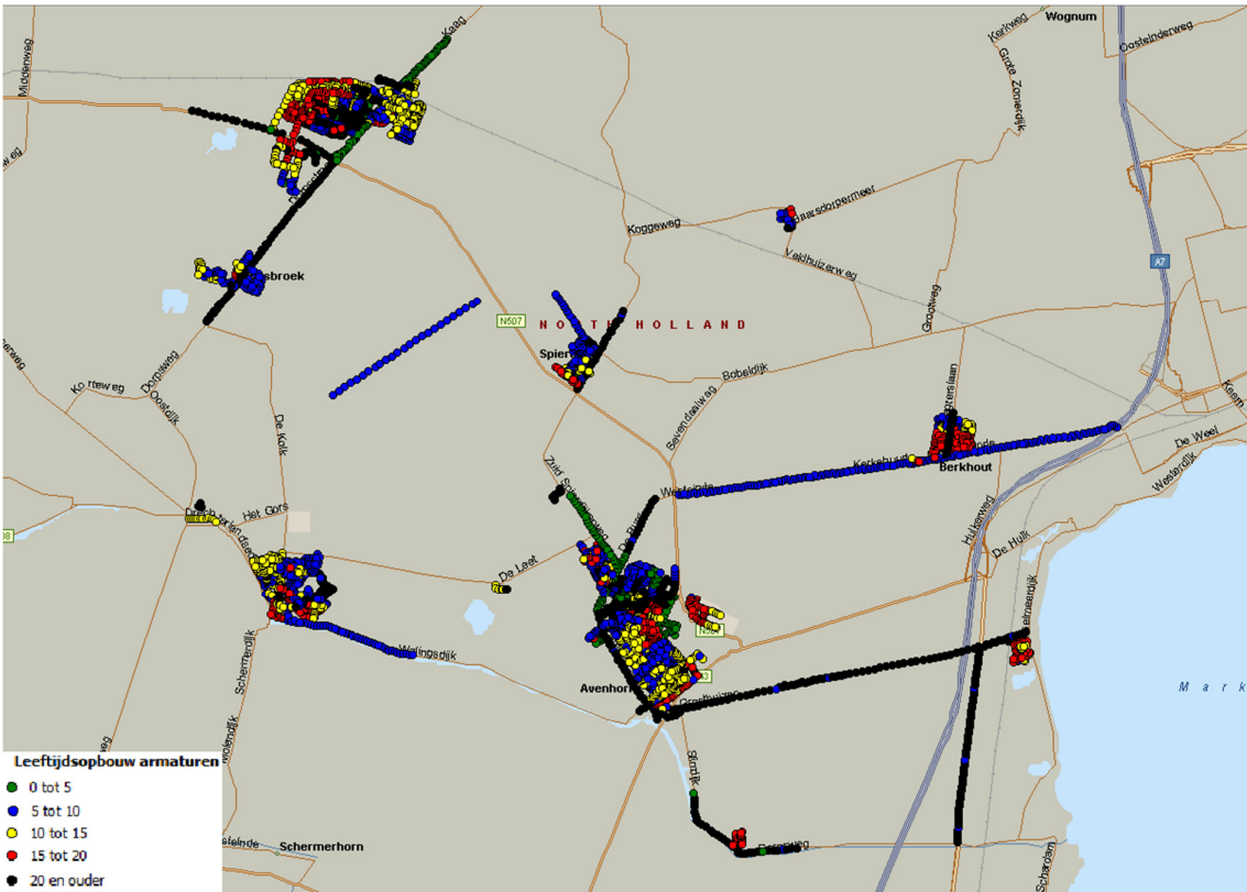
Figuur 5: Totaaloverzicht leeftijdsopbouw armaturen in de gemeente Koggenland
