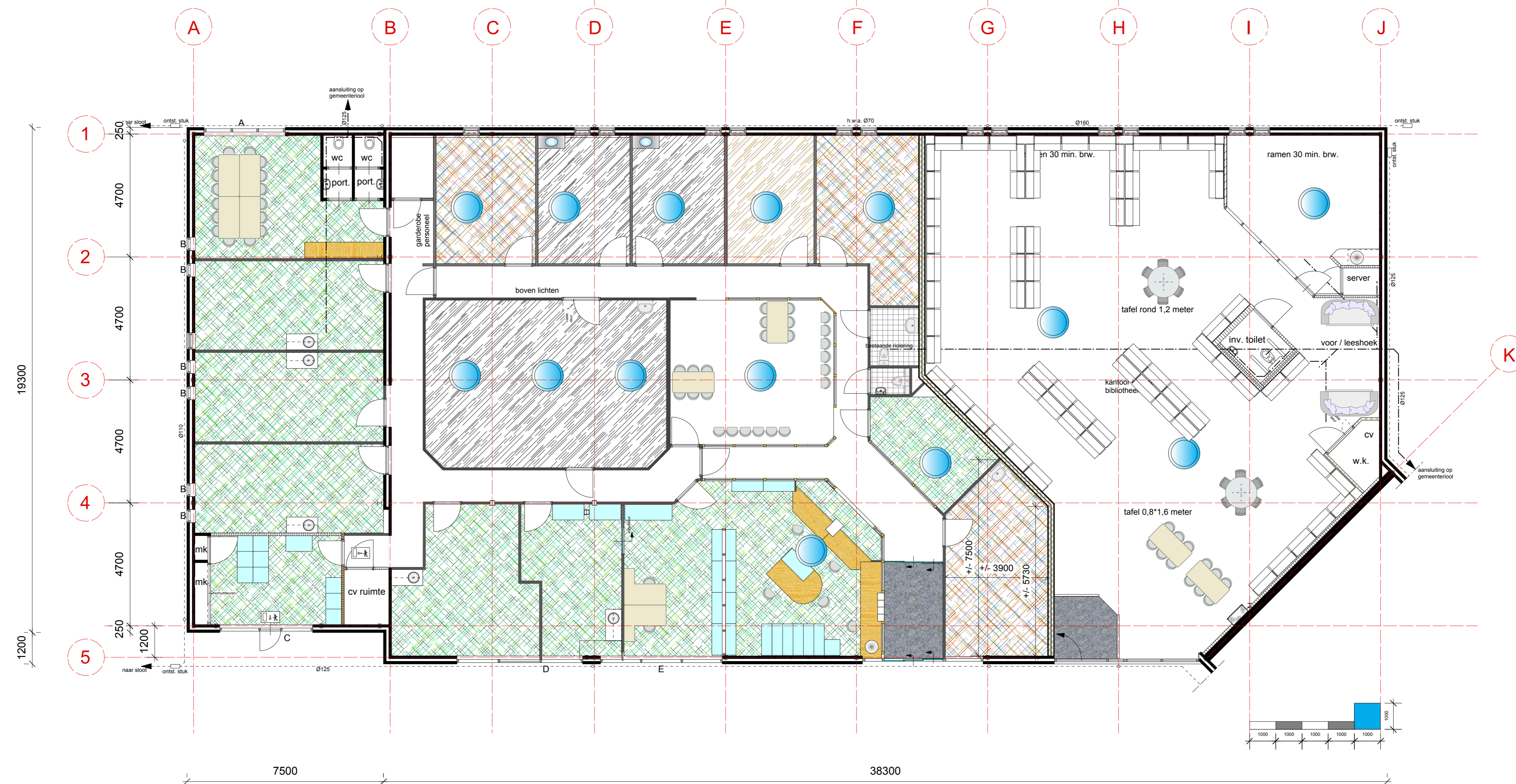
Schets 10 C Transitie Dwingel 3 tot praktijkruimte en bibliotheek met eigen entree Gemeente Koggenland d.d 18-09-2015 schaal 1: 100 A.C.L. Hertog architect HBO
