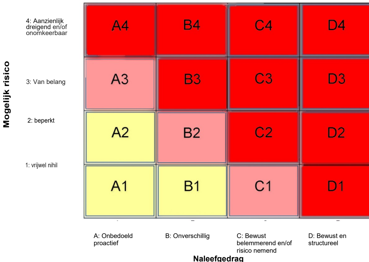
Figuur 2. interventiematrix
